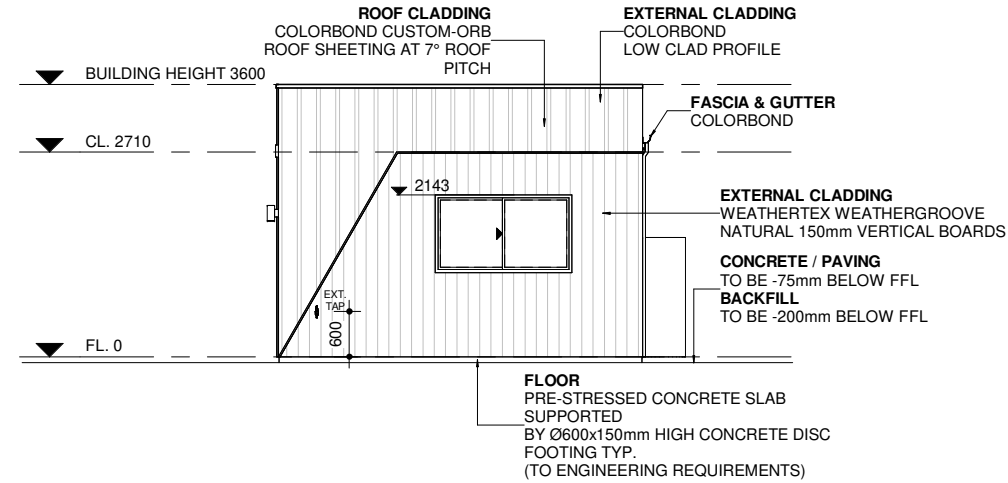
E4 E4 ELEVATION A103 1 : 100
